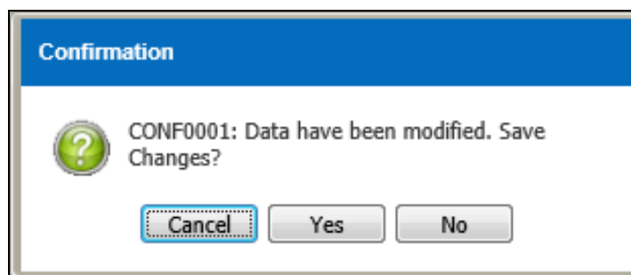
Figure 3.4.2-4 Confirmation Message
