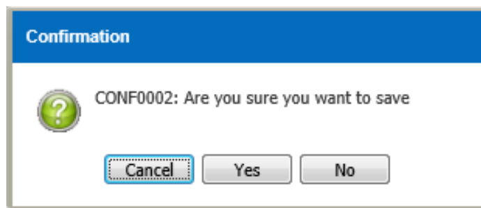
Figure 3.4.1-5 Confirmation Message
